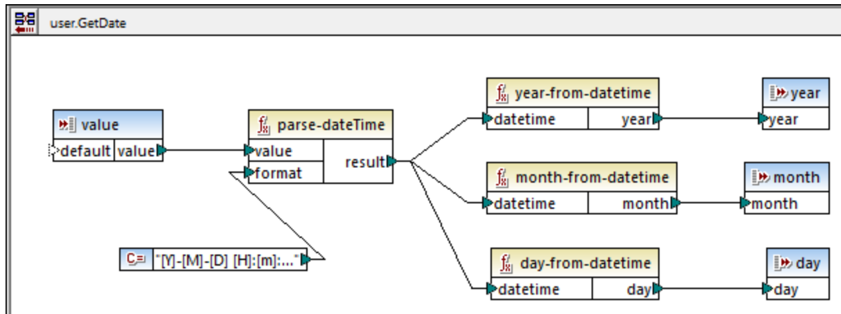
Función definida por el usuario "GetDate"
