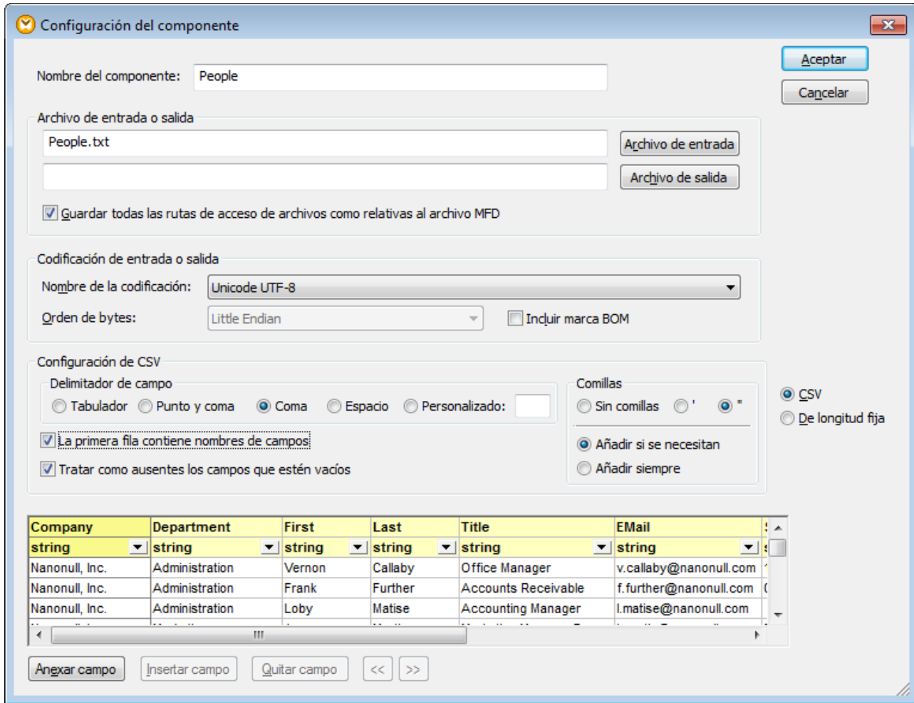
Cuadro de diálogo "Configuración del componente" (en modo CSV)
