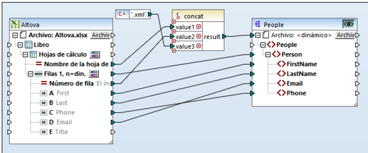
ConvertExcelRows.mfd (segunda parte)
