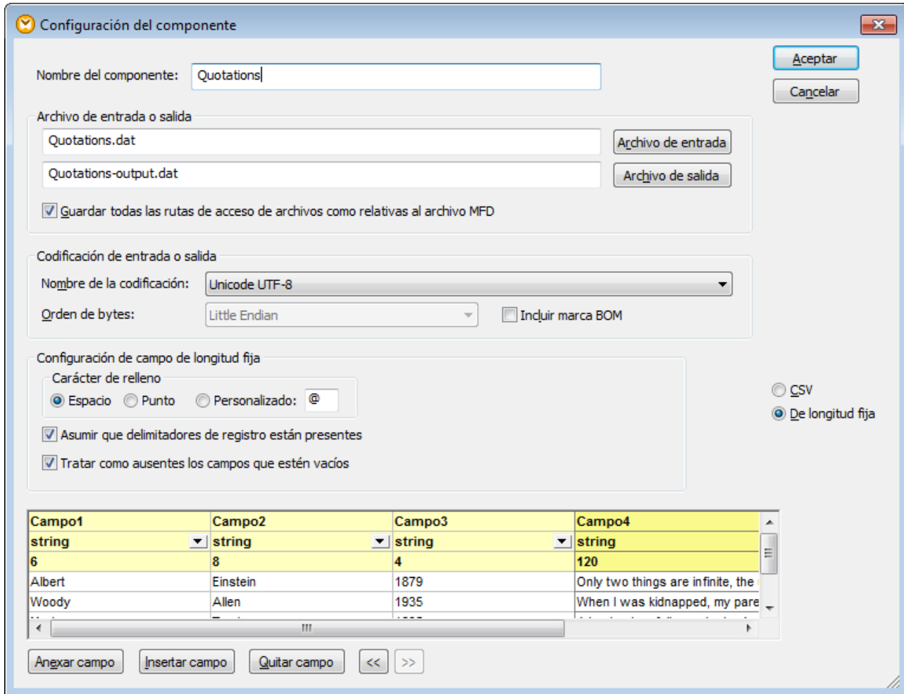
Cuadro de diálogo "Configuración del componente" (en modo de longitud fija)
