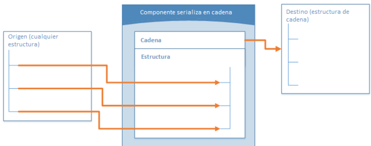
Componente de serialización de cadena genérico
