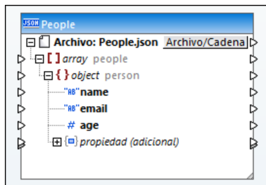
Componente JSON en MapForce
