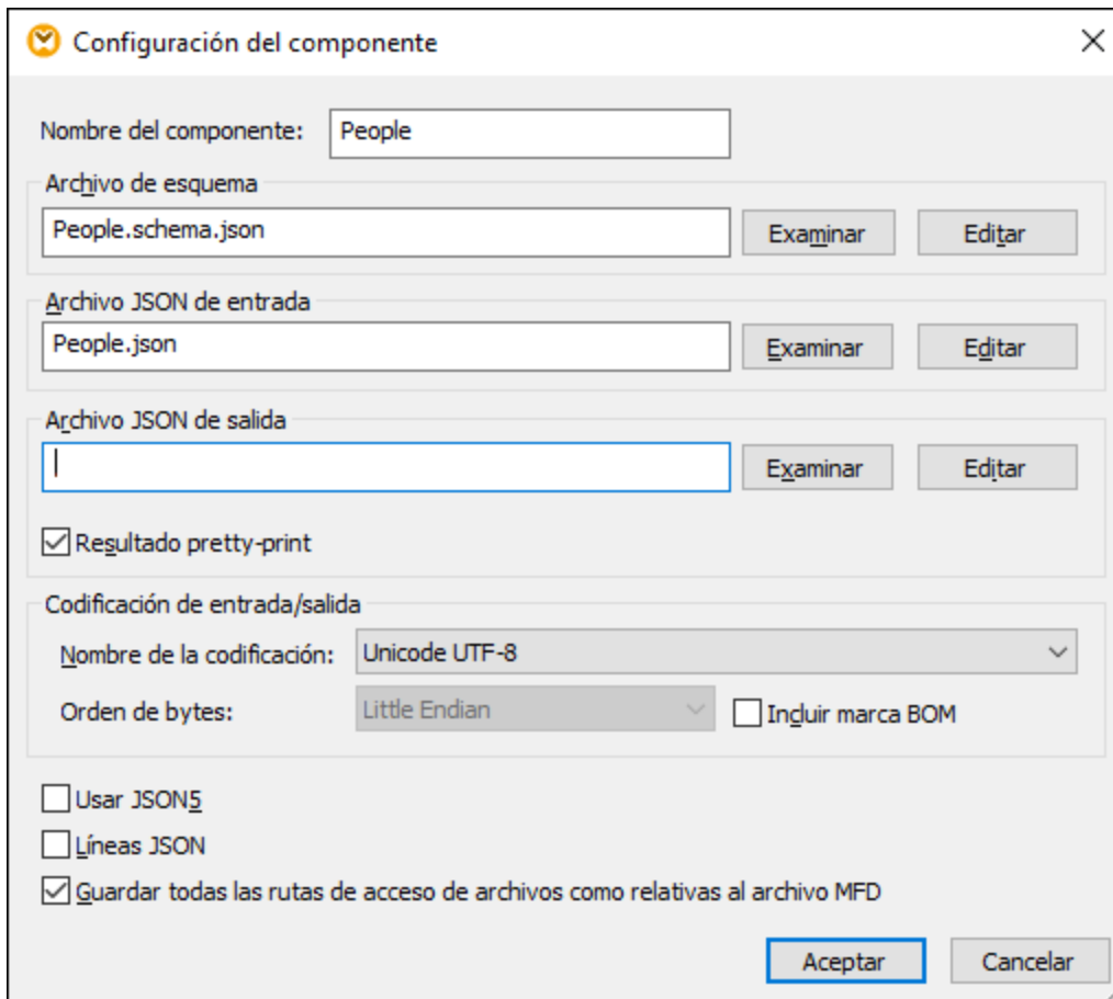
Cuadro de diálogo "Configuración del componente"
