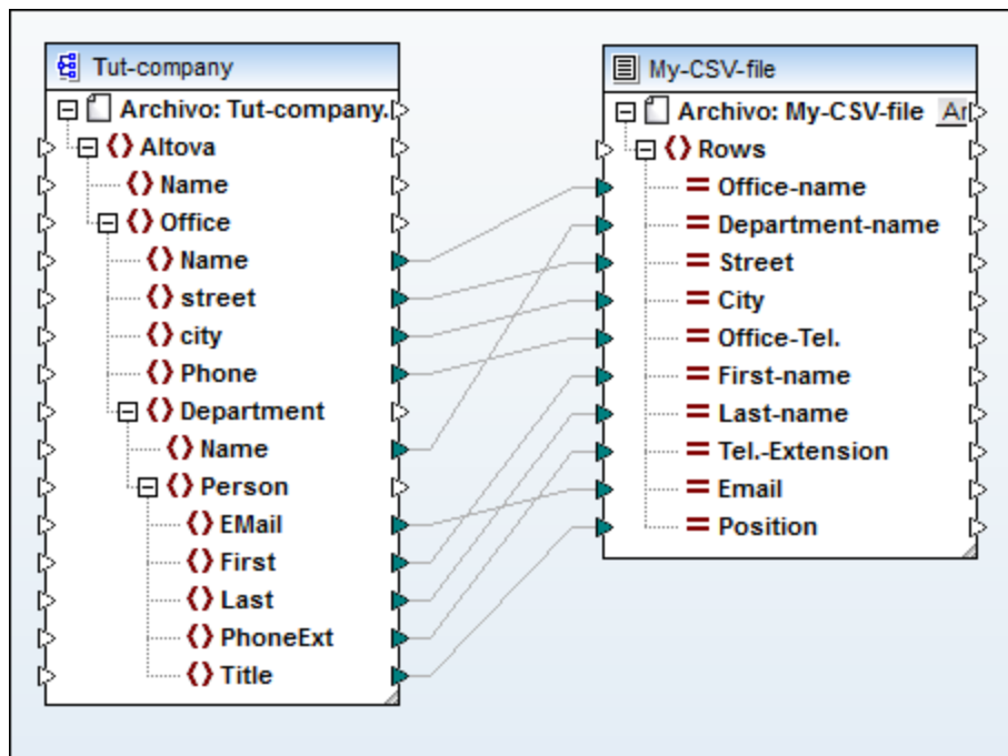
Tut-xml2csv.mfd
