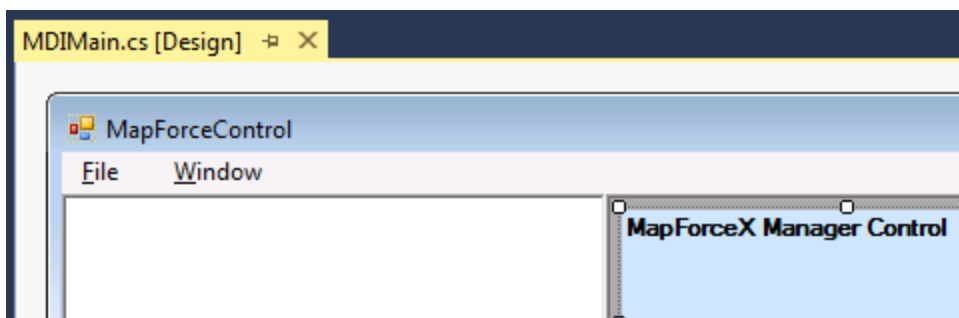
MDIMain.cs
