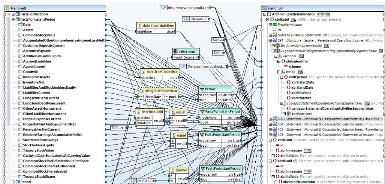
Asignación DB_to_XBRL.mfd
