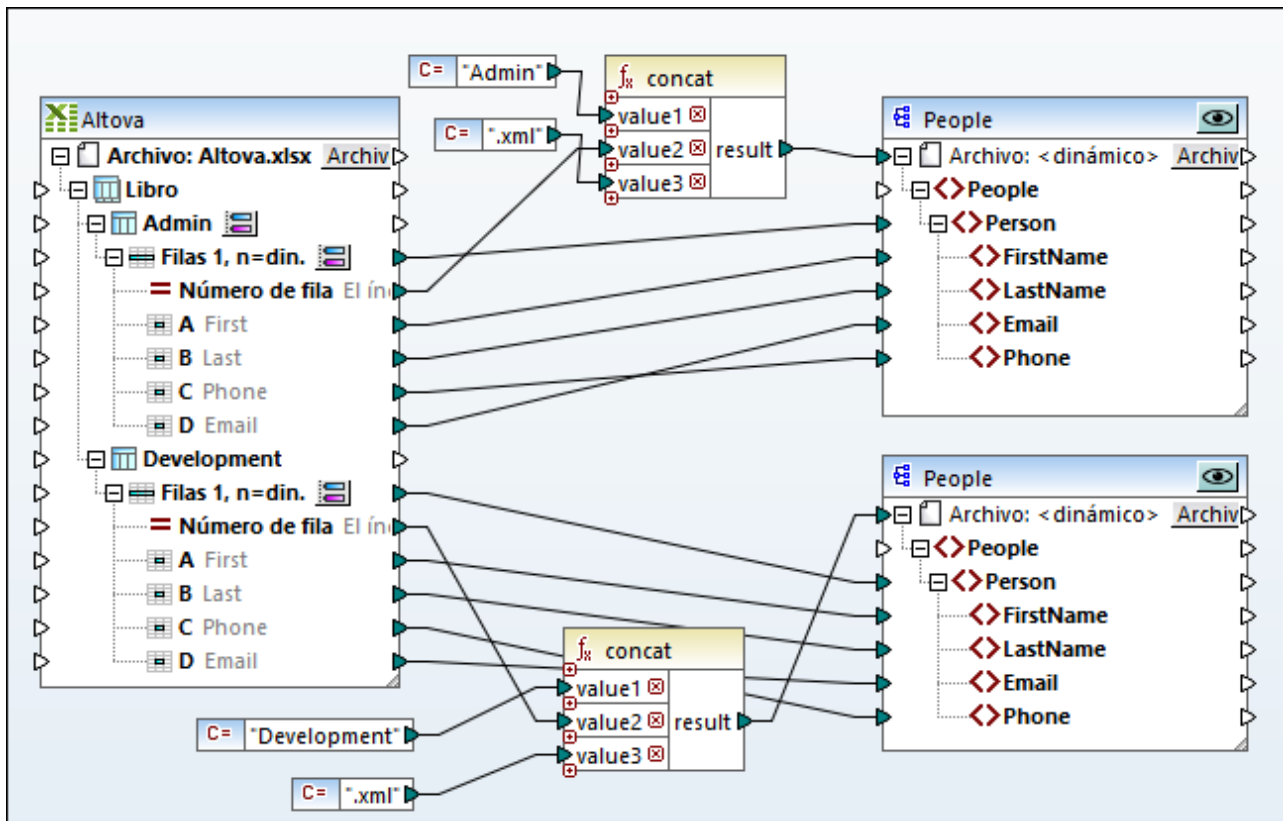
ConvertExcelRows.mfd (primera parte)
