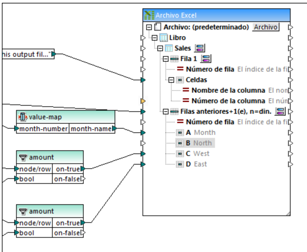
Sales_to_Excel.mfd mapping (después de los cambios)
