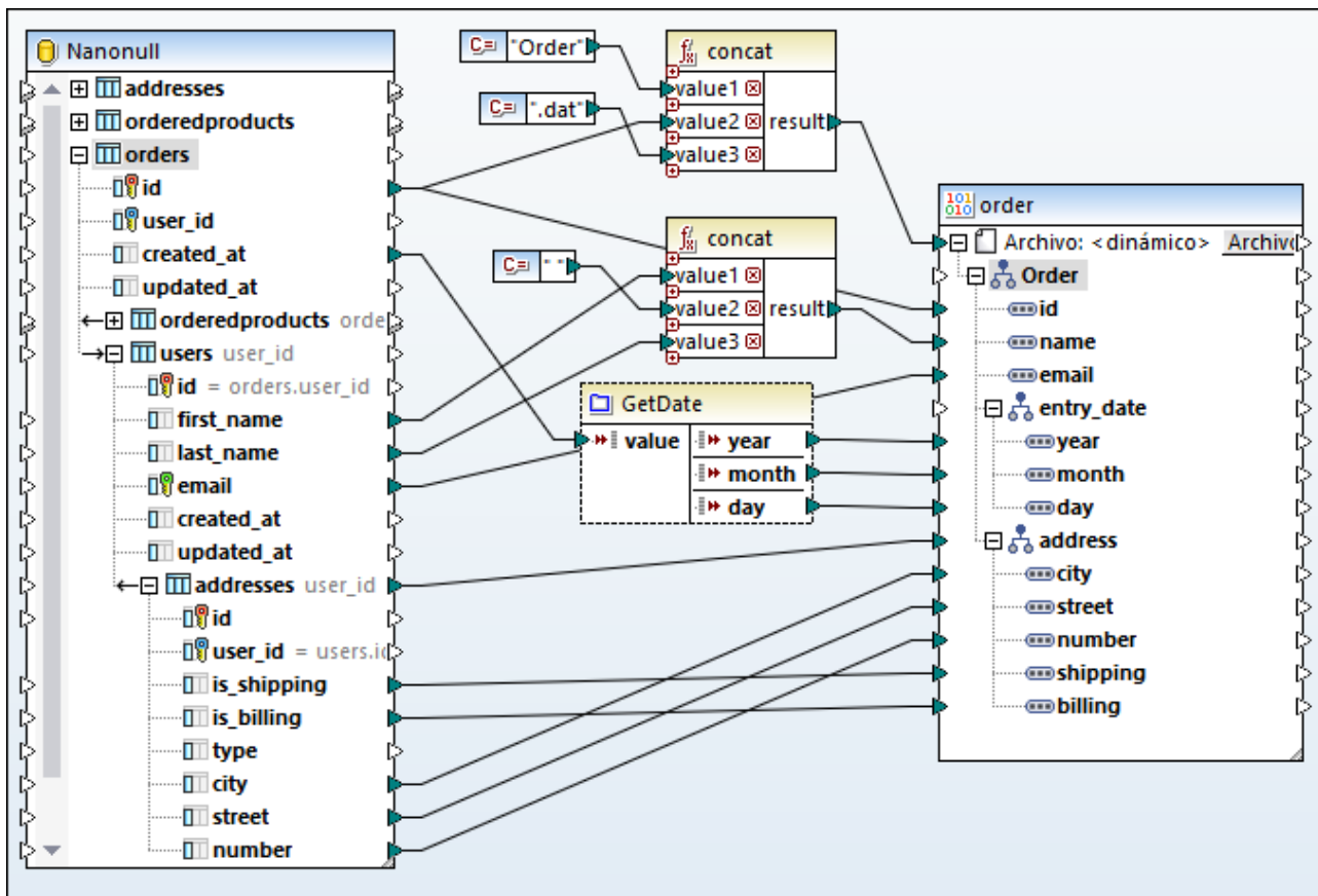
GenerateOrders.mfd
