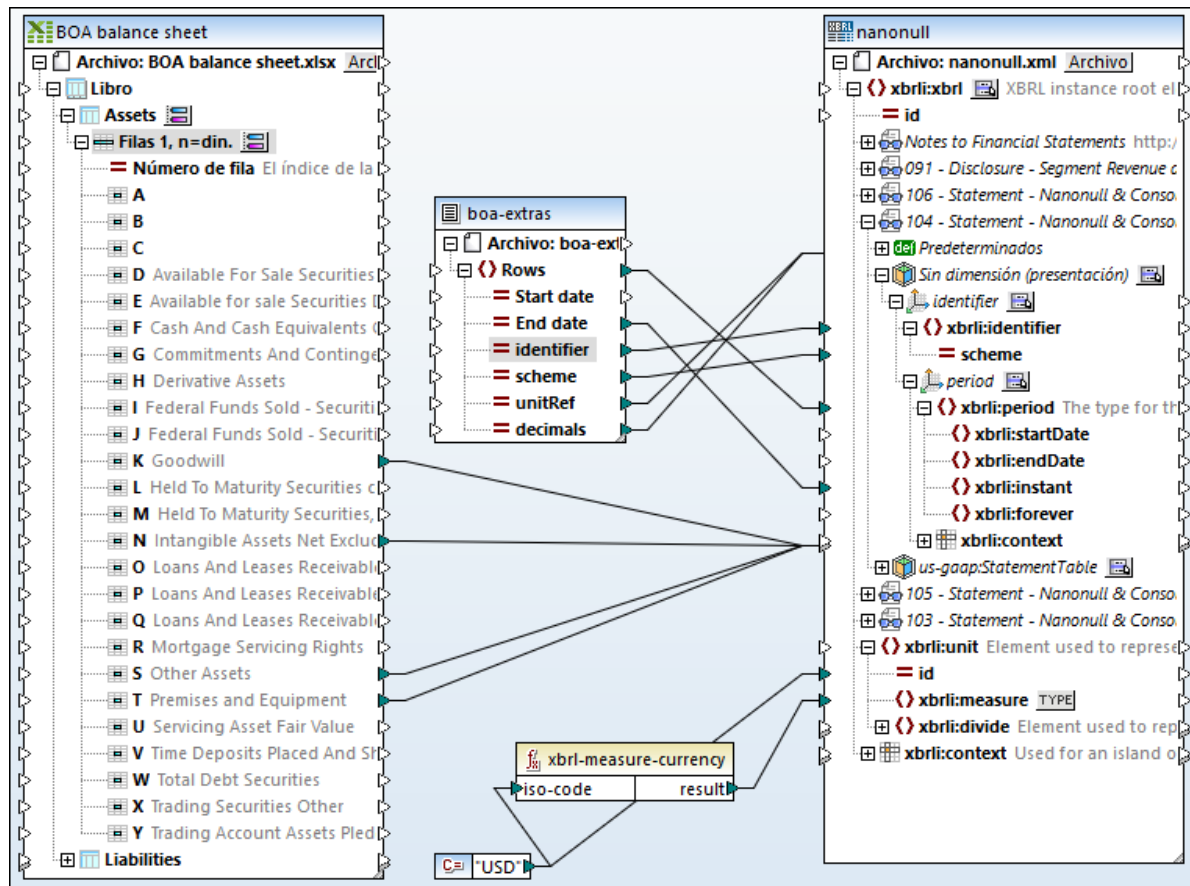
Asignación boa-balance-sheet.mfd
