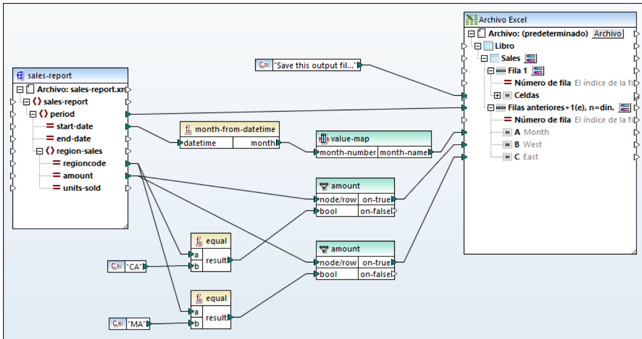
Sales_to_Excel.mfd
