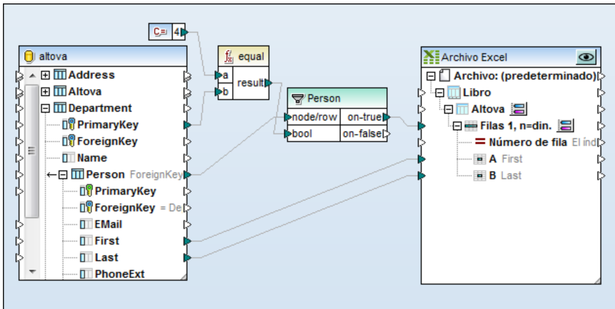
Excel-mapping.mfd (ejemplo nº3)
