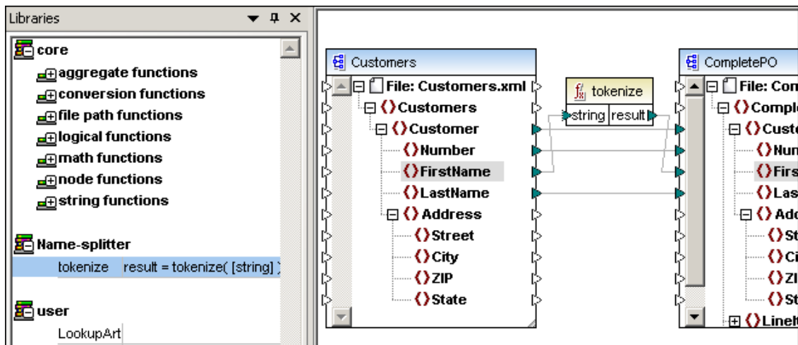
XSLT ausgewählt
