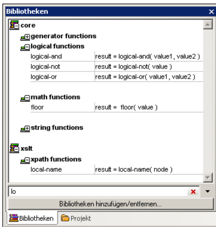
XSLT ausgewählt
